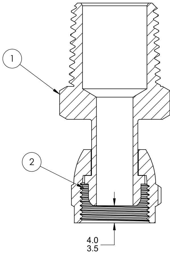
SECTION A-A
