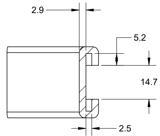
SECTION AJ-AJ
