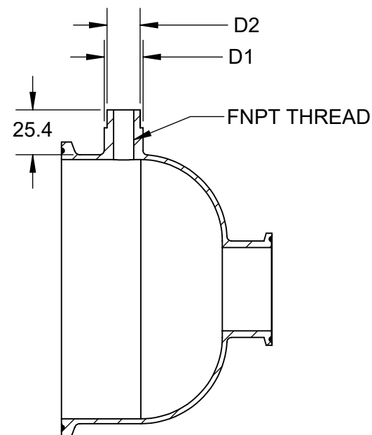
SECTION BA-BA SCALE 1 : 3
