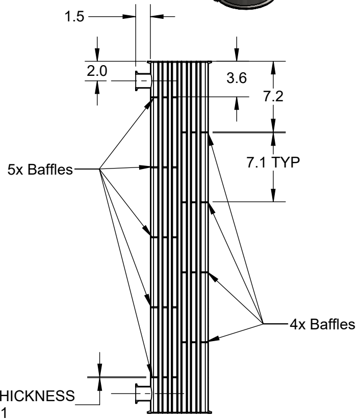
SECTION A-A
