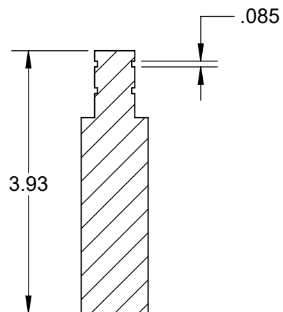
SECTION D-D
